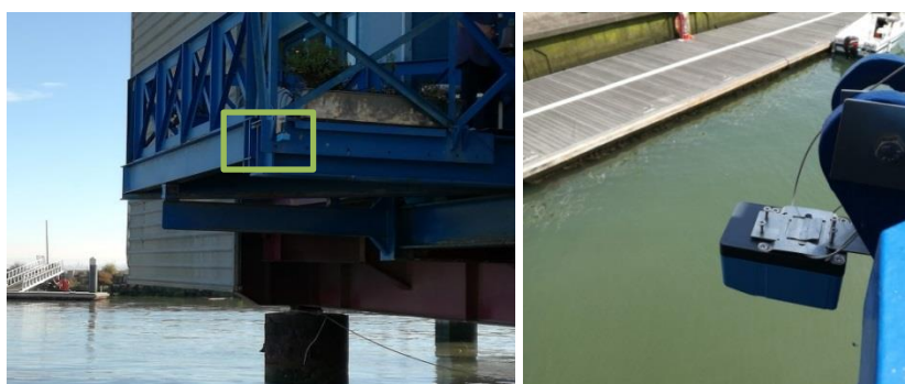
Figure 4.13 – General overview of the sensor SenZ2 installed in the Parque das Nações Marina
